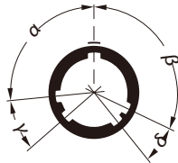
插座正视图
